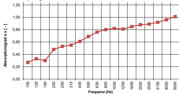
Schallabsorptionsgrad nach DIN EN ISO 354, DIN EN ISO 11654, ASTM C 423
