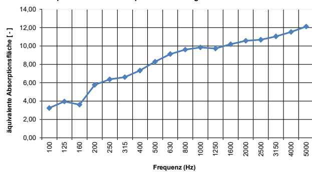
äquivalente Schallabsorptionsfläche der ganzen Fläche
